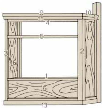
書院部材セット「銀杏」の組立図
