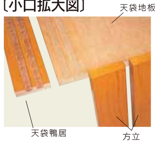
〔小口拡大図〕
